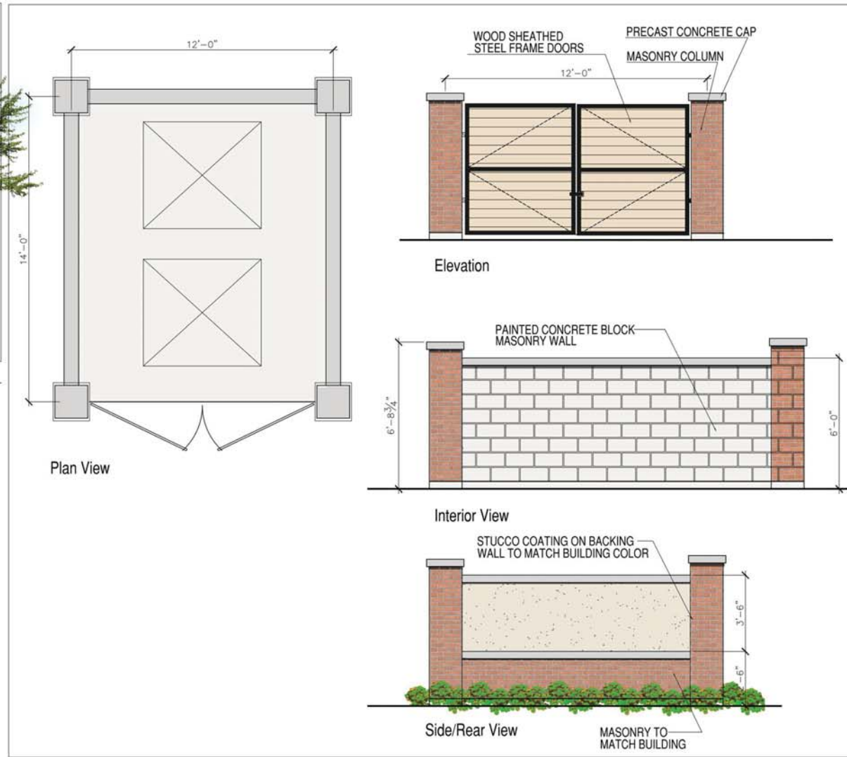
Trash Enclosure Scale: 1/2"=1'-0"
